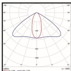
LDC polaire
