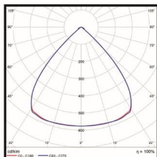
LDC polaire
