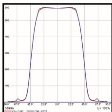
LDC linéaire
