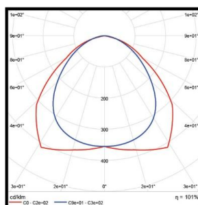
LDC polaire
