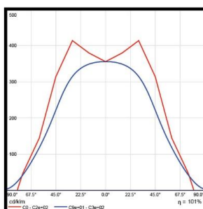
LDC linéaire
