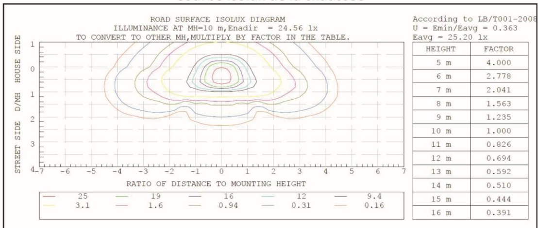
Courbe Isolux de la chaussée
